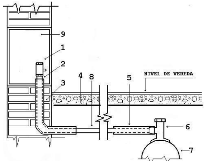
Imagen N° 4.- Servicio domiciliario.
