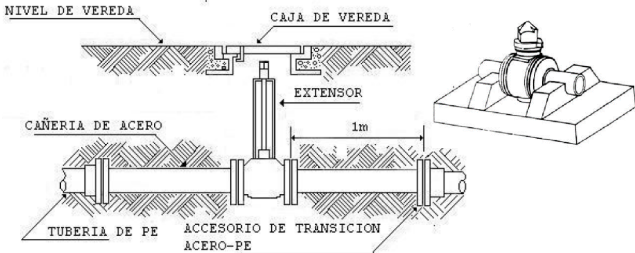
Imagen N° 3.- Válvulas.
