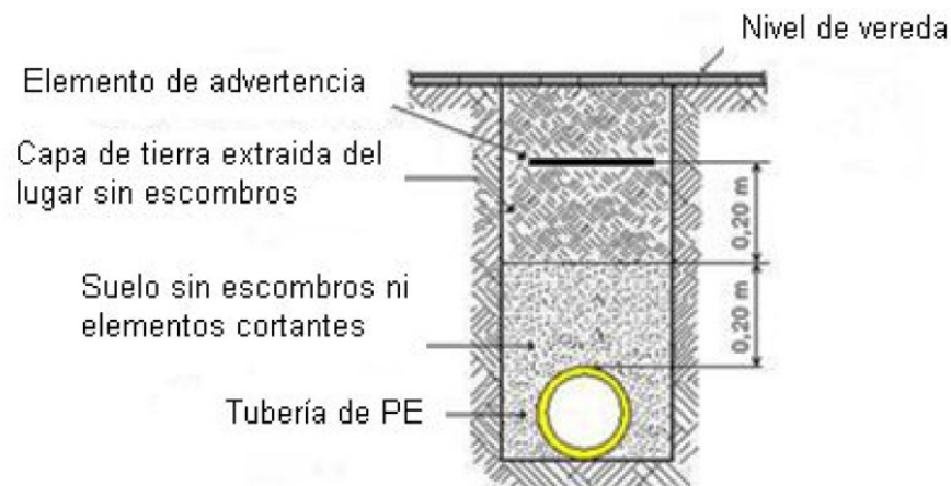
Imagen N° 1.- Tapadas mínimas.
